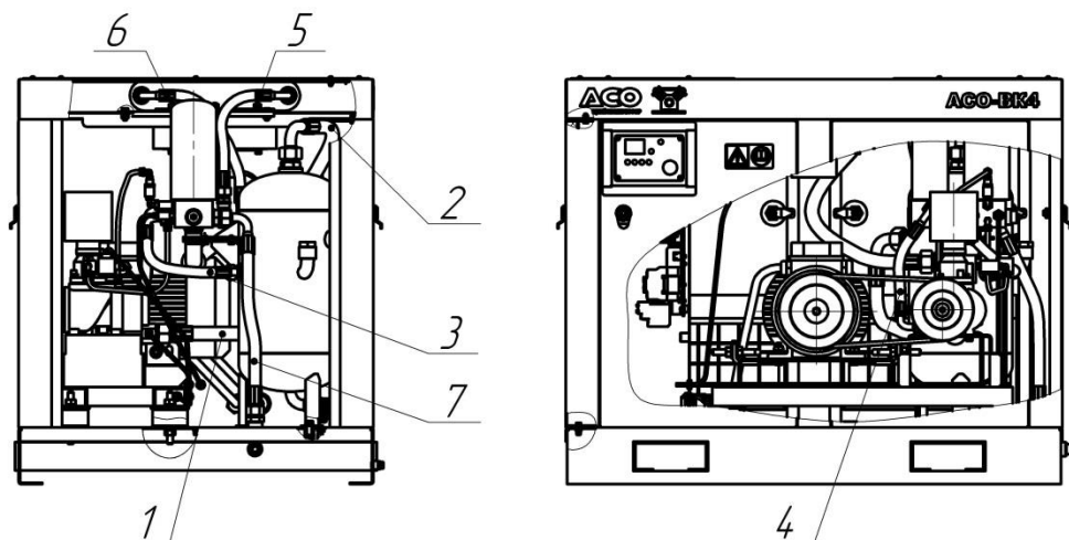
Рисунок 10 – Схема расположения рукавов Таблица к схеме расположения напорных рукавов
