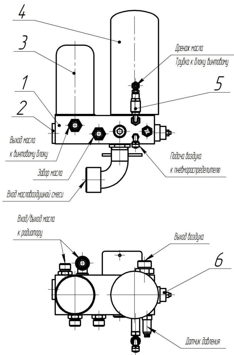
Рисунок 7. Мультиблок
